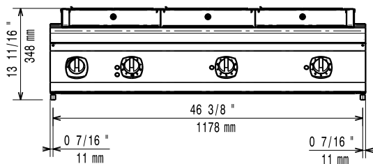
Alzado
